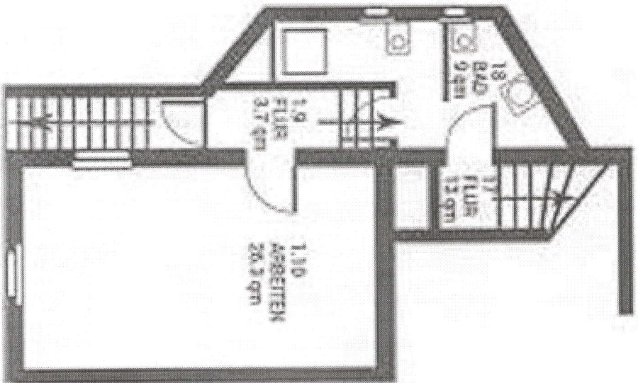
UNTERGESCHOSS
